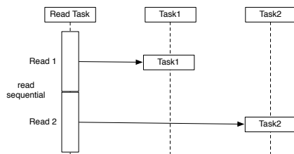
図 6 Read Task と WordCount の分離
