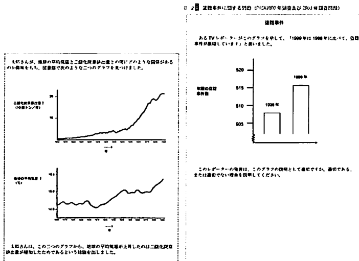
図3 PISA 問題例 9) 。左は相関関係と因果関係の違い、右は省略棒グラフ。
