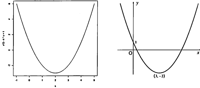
図1 左: curve(x^2-4*x+1, xlim=c(-1,5)) の出力。右: 右のような高校数学の教科書風のグラフにするためには少し工夫が必要である(「統計・データ解析」サイト 6) の「グラフの描き方」参照)。
