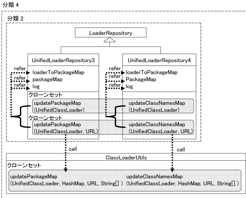
図 14 分類 4 のチェンドクローンセットの例 Fig. 14 Example of Category 4.
