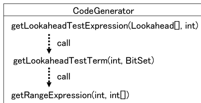
図 11 図 10 のチェンドクローンセットをリファクタリングした例 Fig. 11 Example of refactoring of a chained clone set of Fig. 10.
