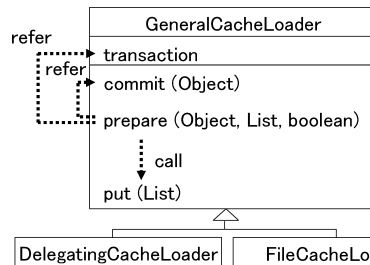
図 13 図 12 のチェンドクローンセットをリファクタリングした例 Fig. 13 Example of refactoring of a chained clone set of Fig. 12.
