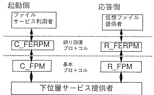
図 6: FTAM の機能モデル
