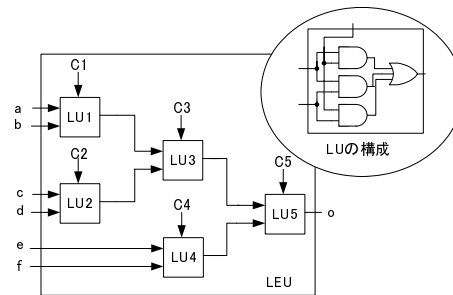
図 4 LEU の構成図
