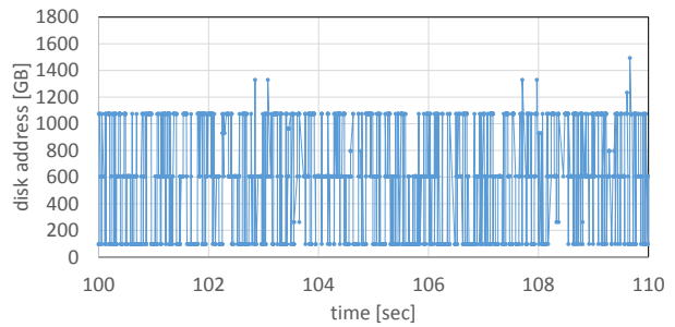
図 4 2DB(tuned) 新規ノードのディスクアクセス
