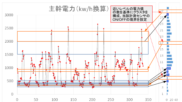
図 6 電力量値の離散レベル値変換手法の概要
