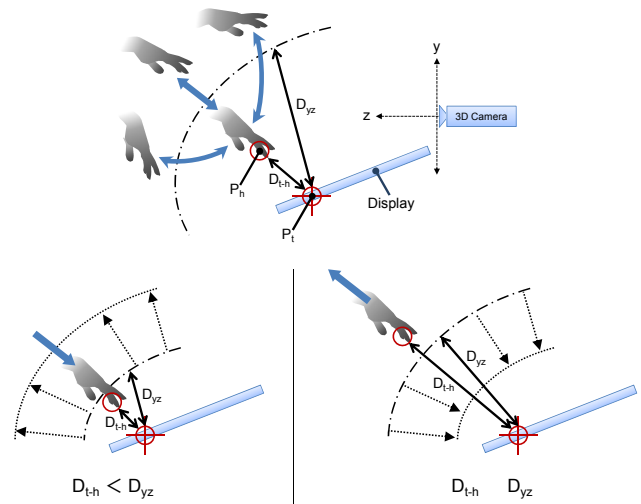
図4 手の近づきの認識アルゴリズム Fig. 4 Recognition Algorithm of Closing a Hand.
