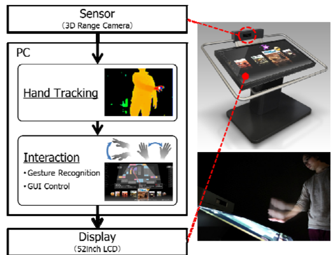
図 7 プロトタイプの構成
