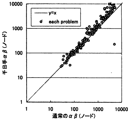
図6 3×3における千日手判定の有無による比較
