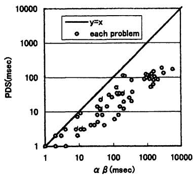
図5 3×4における \alpha\beta とPDSの計算時間の比較 表3・表4は、PDSの成れる段による解けた数とノード数の比較である。本将棋の成段は「3」で、
