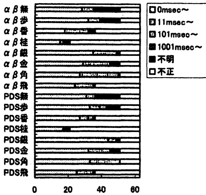
図3 3×3における駒の有無による結果の分布
