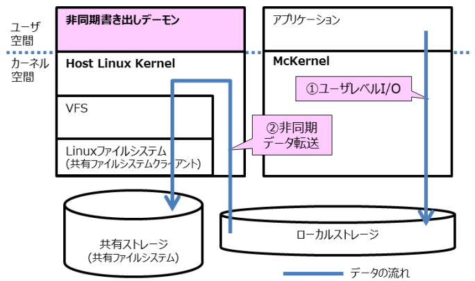
図 5 ユーザレベル I/O と非同期データ転送の流れ
