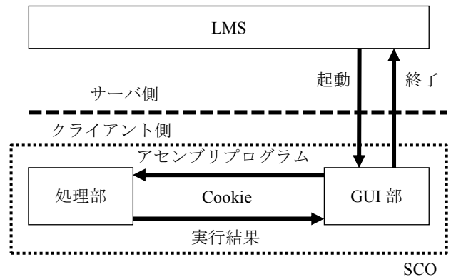
図 7 SCORM パッケージのモジュールとデータの流れ Figure 7 Modules and Data Flows in the SCORM Package.
