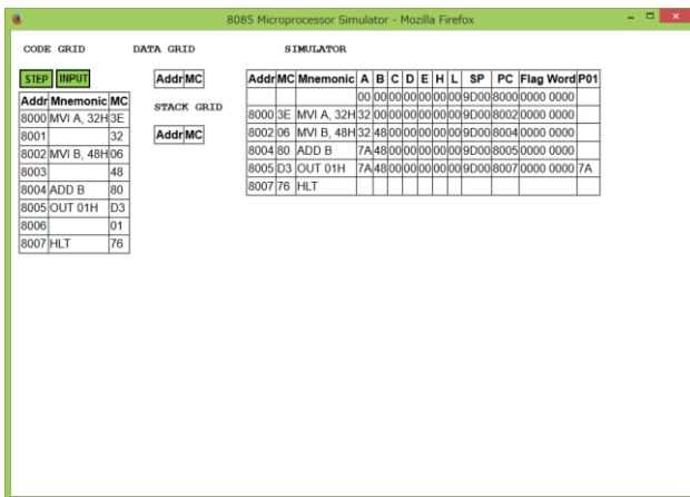
図 3 アセンブリプログラムの出力画面 Figure 3 Output Window of an Assembly Program.
