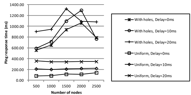
図 10 Ping の平均応答時間
