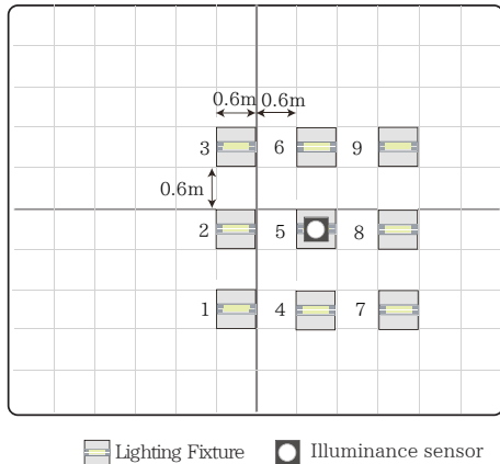
図 3 照度センサの特性調査実験環境
