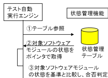
図2 状態管理テーブルと連携した判定シーケンス Fig. 2 Judgment sequence with state management table
