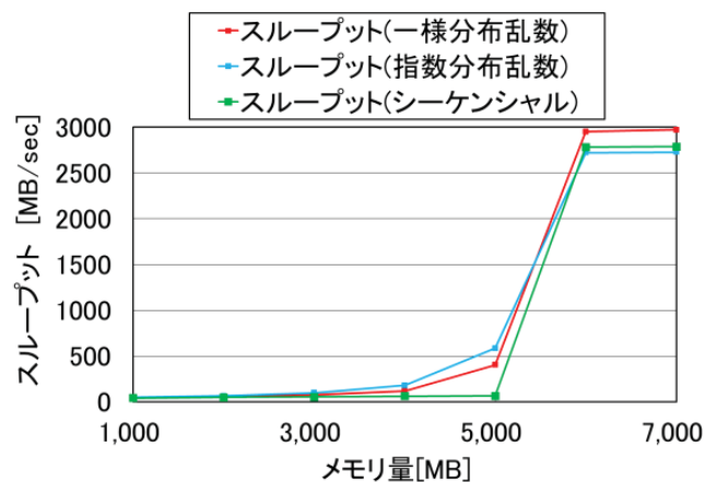
図2 スループットの測定
