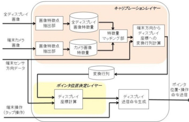
図 2 提案システム構成図
