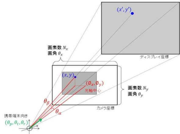
図4 ディスプレイ・カメラ・携帯端末方向の幾何関係
