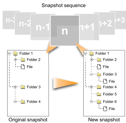
(a) スナップショットの再構成
