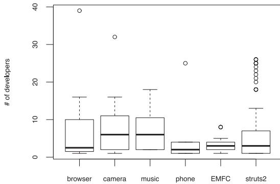
図 5 クローンセットのメソッドを変更した開発者数
