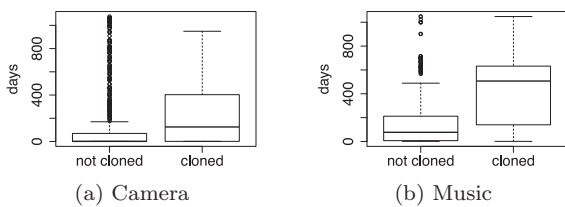
図 4 クローン有無とメソッドの存在日数
