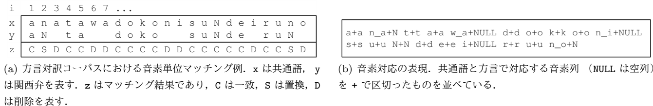
図 2 音素変換ルールの基本的なアイデア.
