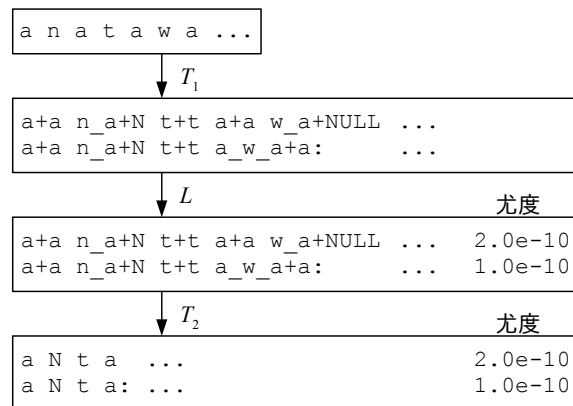
図 3 WFST T_1 , T_2 , L の役割.
