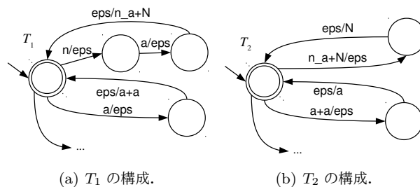
図 4 WFST T_1 , T_2 の構成. 各遷移に対して入出力記号組を / で区切って示した。eps は記号なしでの遷移を示す。
