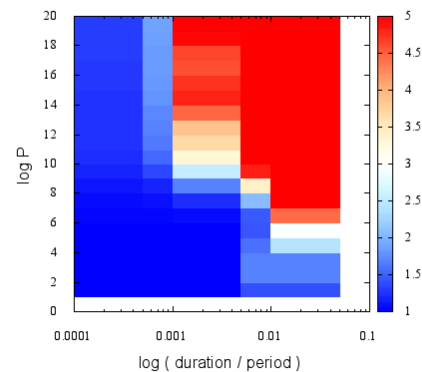
図 18 ジッタの影響 ( z 軸の範囲 [1,5])
