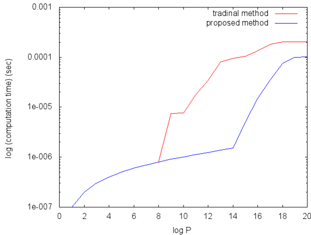
図 12 従来手法の計算時間と提案手法の計算時間の最小値 ( T_{\text{comm}}/\text{duration}=1.0\text{e-}2 , \text{period}=1.0\text{e-}3 , \text{duration}=1.0\text{e-}5 )
