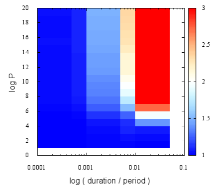
図 14 ジッタの影響 (Z 軸の範囲 [1,3]) (ジッタありの従来手法の計算時間) / (ジッタなしの従来手法の計算時間) ( \text{period}=1.0\text{e-}3 , N=8 )
