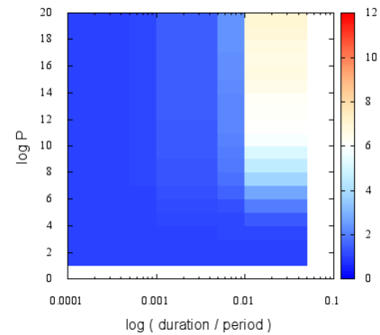
図 13 ジッタの影響 (Z 軸の範囲 [1,12]) (ジッタありの従来手法の計算時間) / (ジッタなしの従来手法の計算時間) ( \text{period}=1.0\text{e-}3 , N=8 )
