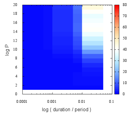
図 17 ジッタの影響 ( z 軸の範囲 [0,80])
