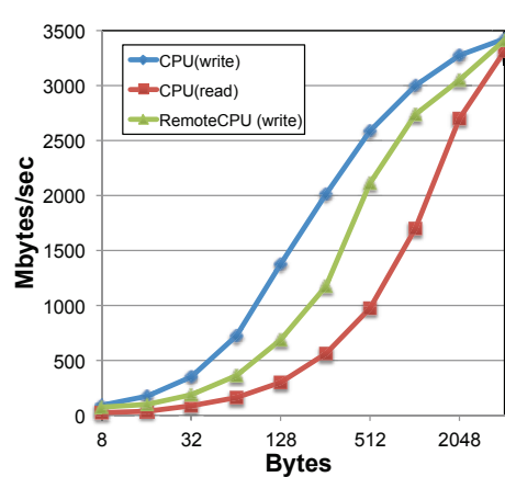
図 9 PEACH2-CPU, 隣接ノード CPU 間の DMA 性能 (255 回連続)
