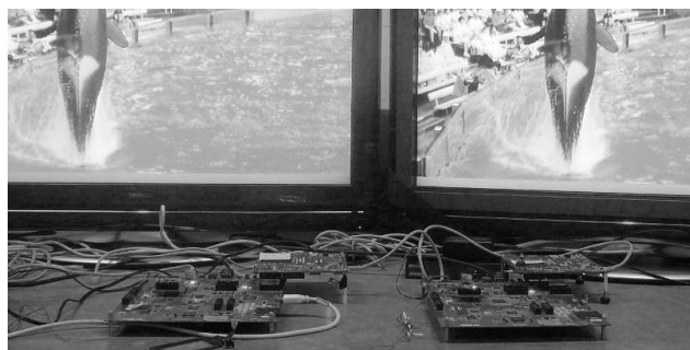
図 10 H.264 コーデックプラットフォームによる実機検証 Fig. 10 H.264 Codec platform testing the algorithm.
