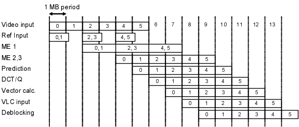
図 1 エンコーダパイプライン Fig. 1 Encoder pipeline example.
