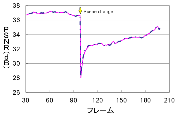
図 12 シーンチェンジ時の PSNR 比較結果 (Square Garden) Fig. 12 Effect on PSNR at scene change. (Square Garden)
