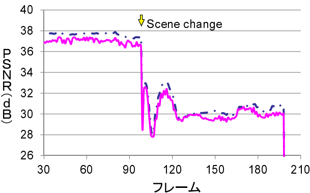
図 14 シーンチェンジ時の PSNR 比較結果 (Square-Whale) Fig. 14 Effect on PSNR at scene change. (Square-Whale)
