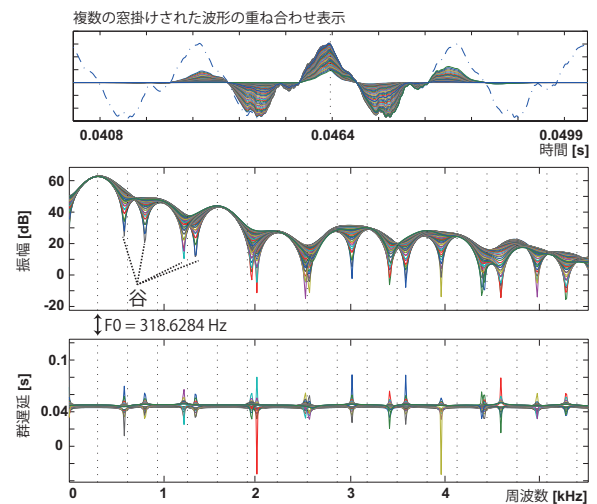
図 3 F_0 に応じた時定数を持つガウス窓を掛けた複数フレームの重畳表示(上図)と、それらに対応するスペクトル(中図)と群遅延(下図)。
