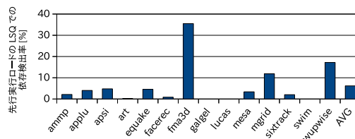
図 1 先行実行 in-flight ロード・ストア間依存検出の割合
