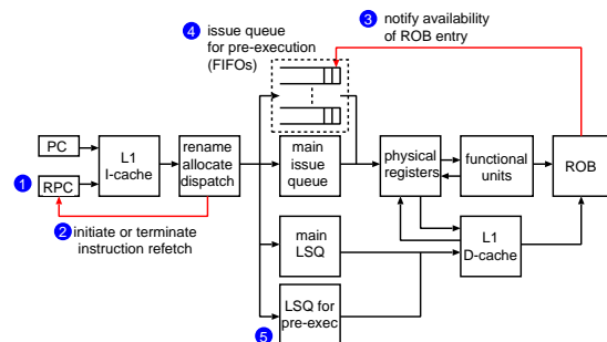
図 2 VROB プロセッサの構成
