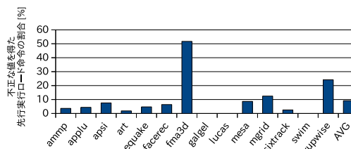
図 7 不正な値を得た先行実行ロードの割合
