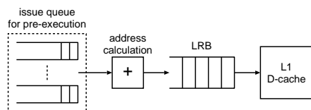
図6 先行実行ロードの処理の流れ
