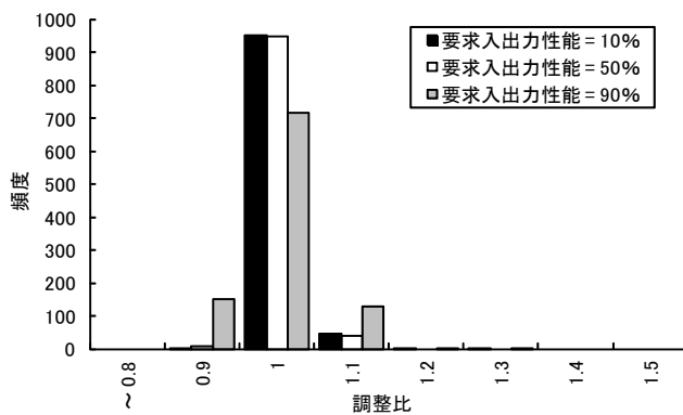
図 5 調整比の頻度分布 (CPU : I/O = 1 : 1)
