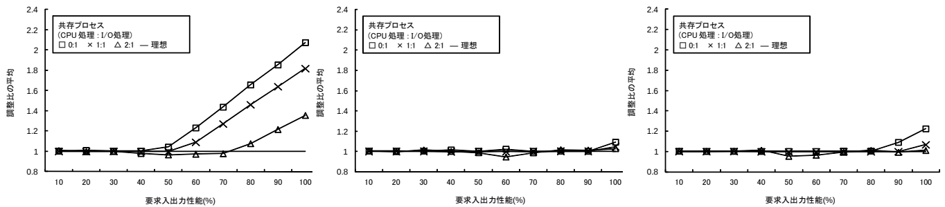
(A) 被調整プロセス (CPU:I/O=0:1) (B) 被調整プロセス (CPU:I/O=1:1) (C) 被調整プロセス (CPU:I/O=2:1)
