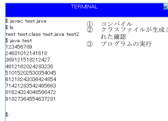
図 5 コマンド実行画面
