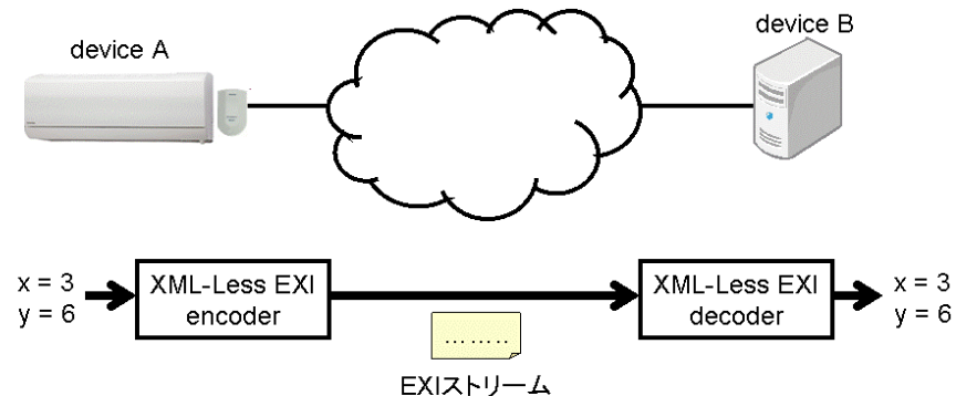
図 3. XML-Less EXI の利用例
