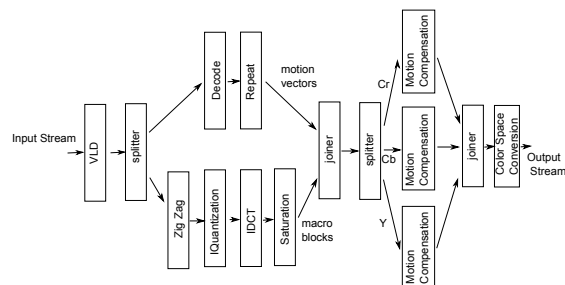
図 1 mpeg デコーダにおけるタスクグラフ Fig. 1 A Task Graph of MPEG2 Decoder System
