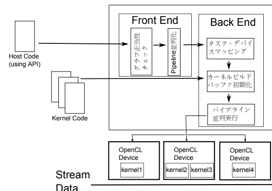
図 6 OpenCL パイプライン並列ライブラリの内部アーキテクチャ
