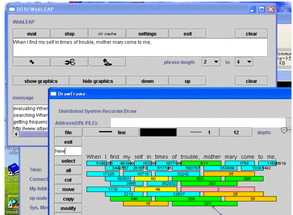
図3. WebLEAP
