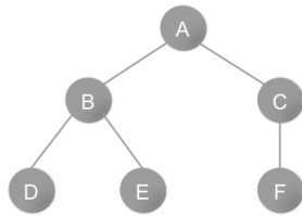
図 1: AST の例
