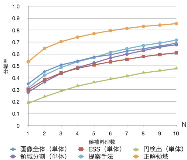
図 8 単品を含む画像での第 N 候補までの分類率
