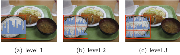
図 5 各ピラミッドレベルで Bag-of-keypoints での特徴ベクトルの作成
