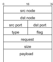
図4 共通パケットフォーマット
