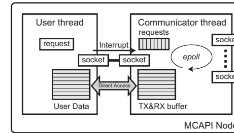
図3 xmcapi/ip の構成
