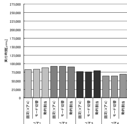
図 11 キャッシュペナルティを除去した実行時間 (5000rpm 時)
