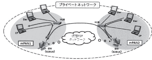
図7 実験環境
