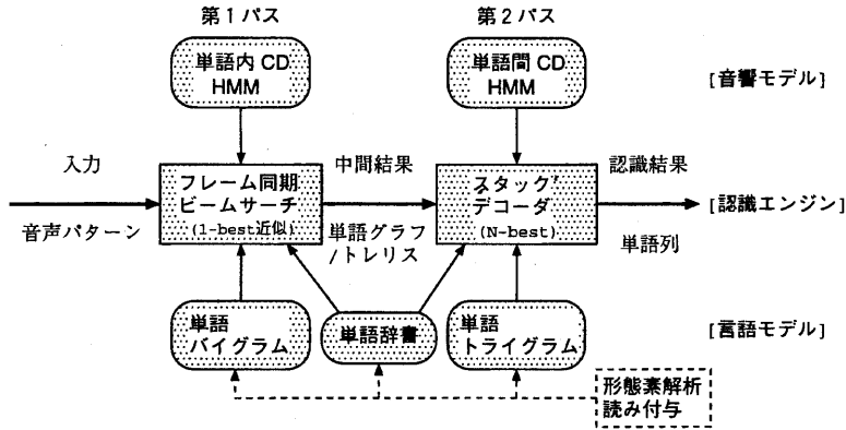
図 2: 日本語ディクテーションシステムの構成
