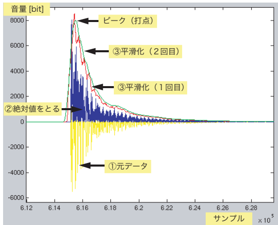
図 4 スネアの打点検出の手順
