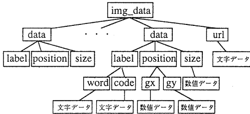
図 3: XML データファイルの構造
