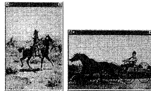
(d) H = 0.82049 (e) H = 0.66194
