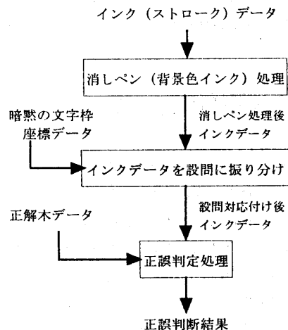
図 4 採点ヘルプ処理
