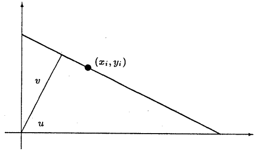
図 1: u-v 変換
