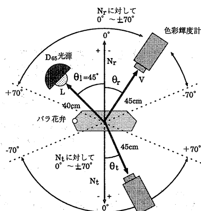
図1: 反射および透過光分布の測定
