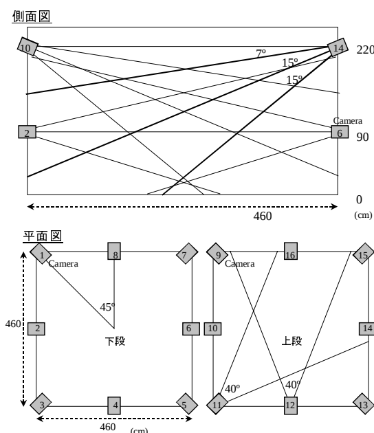
図2. カメラ配置
