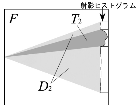
図 6. C_2 における削除可能領域 D_2 の例
