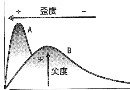
図 3: 尖度と歪度
