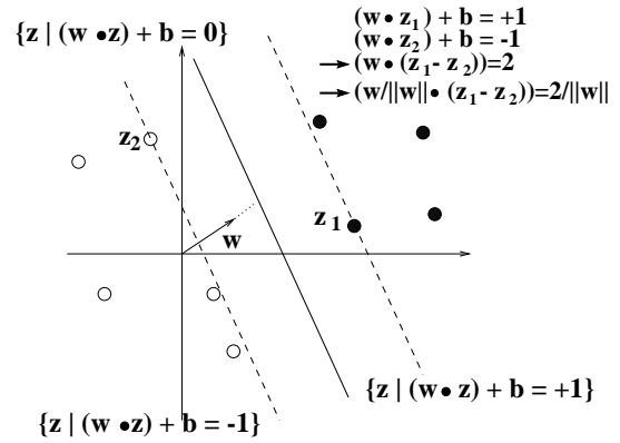
図 1 SVM の例
