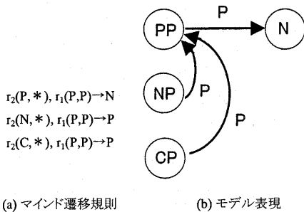
図5 単純でないマインド遷移規則のモデル化
