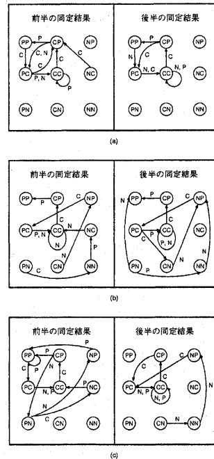
図6 実験1:ユーザのマインド遷移規則の同定結果
