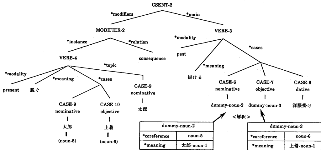
図4. 例文3-1に対する日本語意味構造
