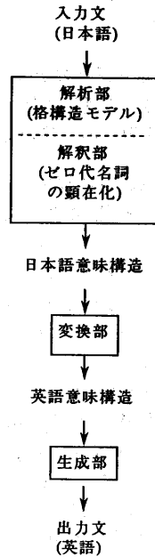
図2. 翻訳処理の流れ
