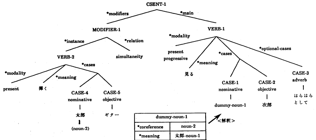
図3. 例文1に対する日本語意味構造
