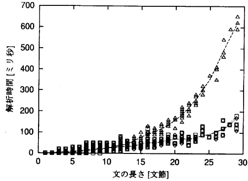
図 5: 文の長さ と 解析時間 の関係
