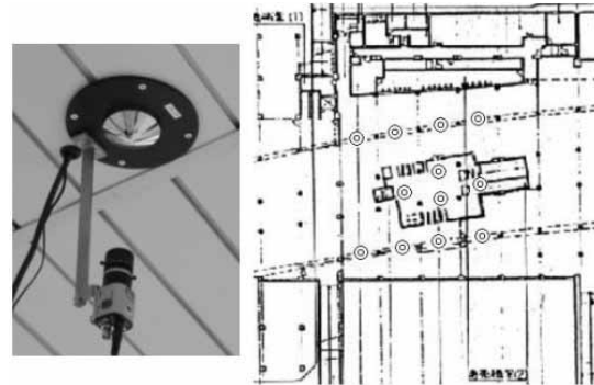
図2：カメラとコンコース階のカメラ配置図
