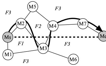
図 2: FACE プロトコル
