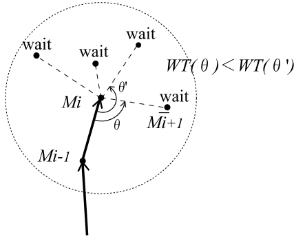
図 4: 待ち時間の設定
