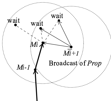
図 5: Prop のブロードキャスト
