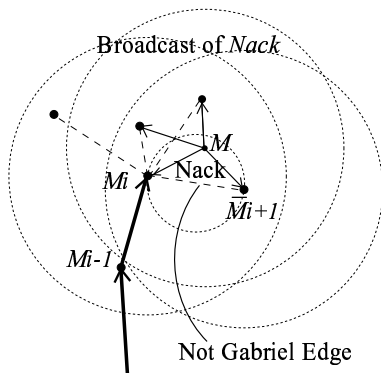
図 6: Nack の送信
