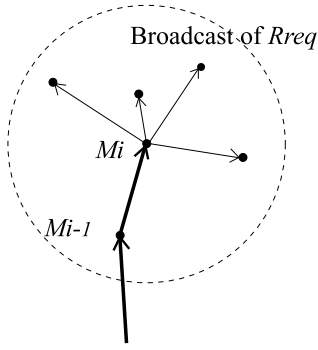
図 3: Rreq のブロードキャスト
