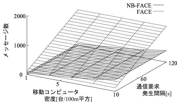
図 8: 制御メッセージ数の比較
