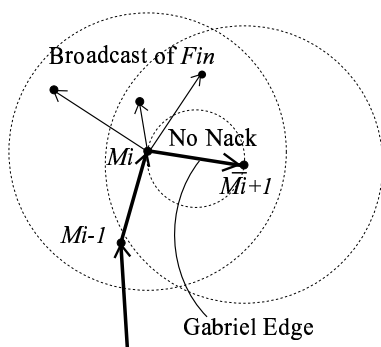
図 7: 次ホップ移動コンピュータの決定
