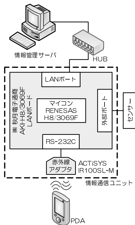
図3 情報通信ユニット (試作機)
