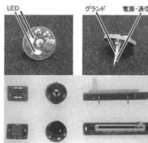
図 3 Pin&Play のデバイス (左からボタン、ダイヤル、スライド)
