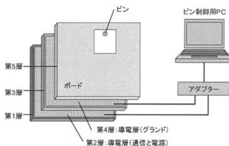
図 2 Pin&Play のシステム構成図
