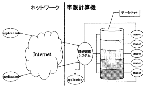
図 2 情報管理システムの概要 Fig. 2 design of information management system
