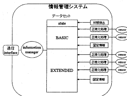
図 5 情報管理システムの実装
